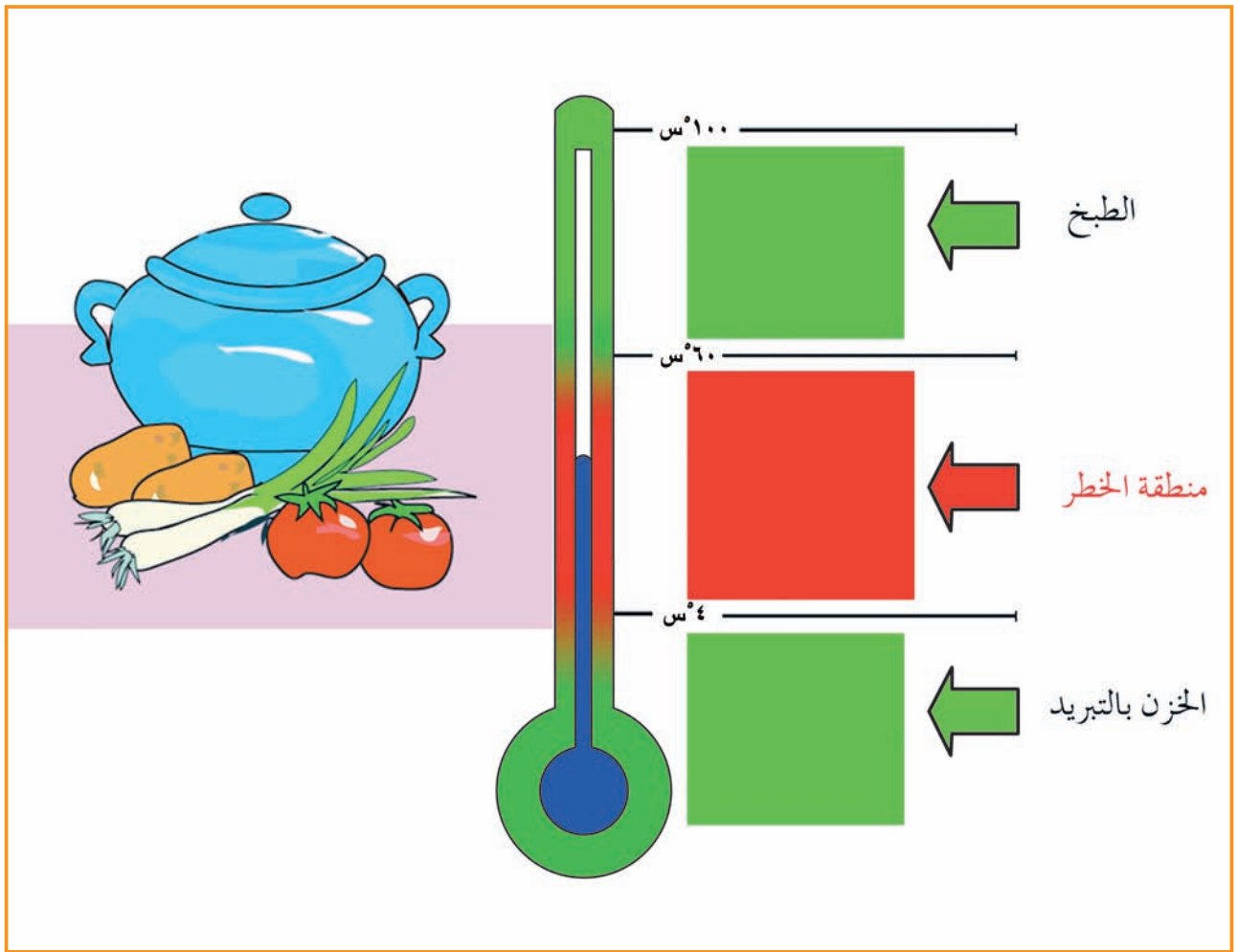
الشكل (٣-٧): درجات الحرارة للسيطرة على البكتيريا في الطعام.
