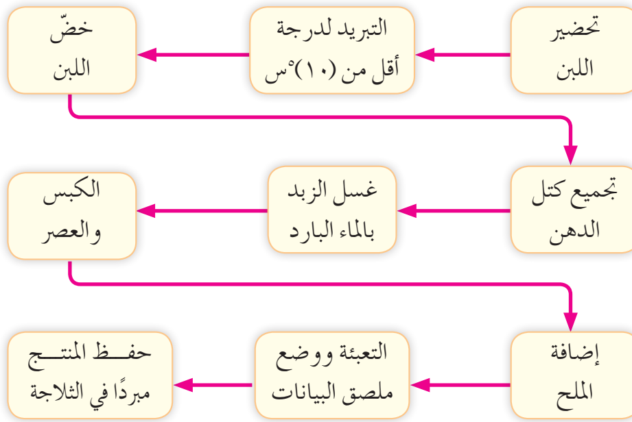
الشكل (٢-٦): مخطط لإنتاج الزبد من اللبن.
